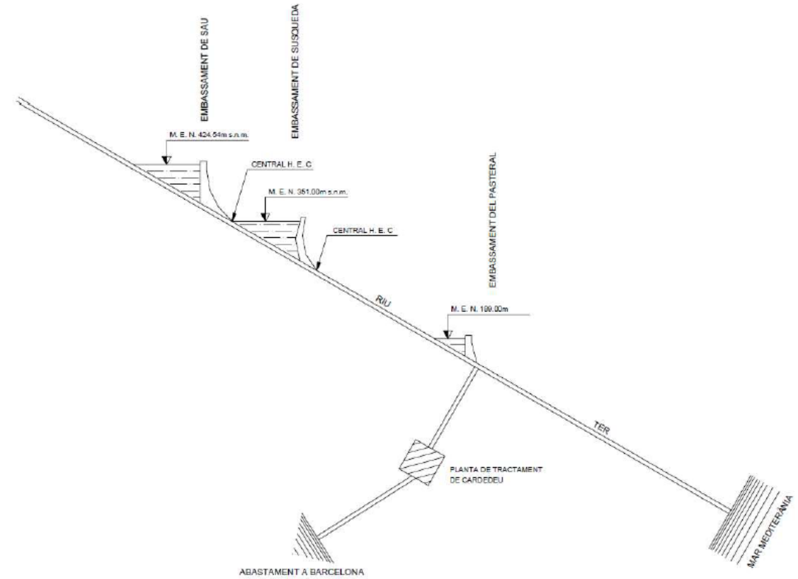
Figura 3. Esquema del sistema Sau – Susqueda - El Pasteral
